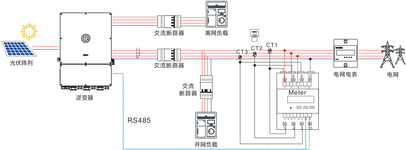
图 5.15. 单个电表系统连接图
