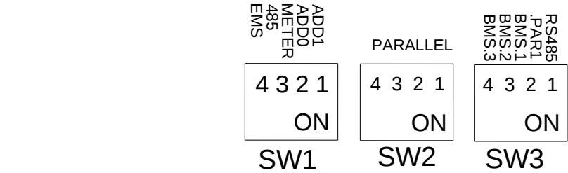
图 5.18. DIP 开关
