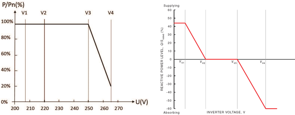
图6.2 电压-有功功率控制曲线（AS4777系列） 电压-无功功率控制模式曲线（AS4777系列）
