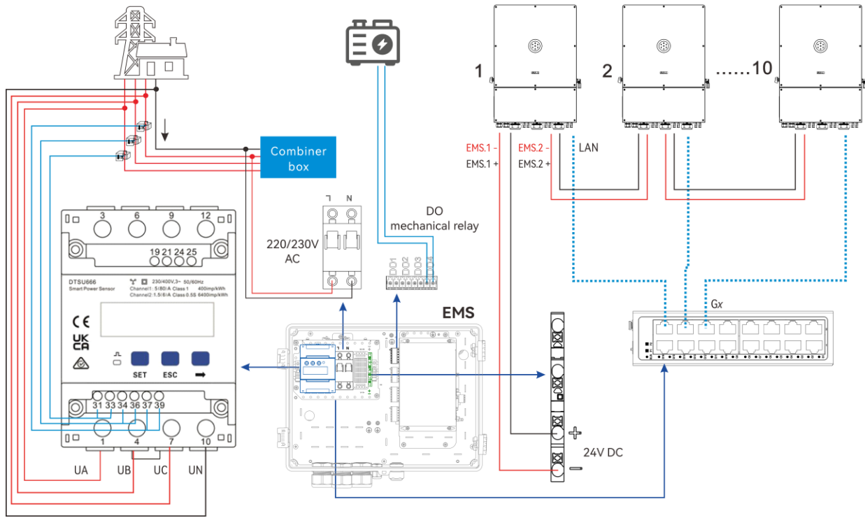
图 5.41. EMS 电缆连接在并机部署中的示意图
