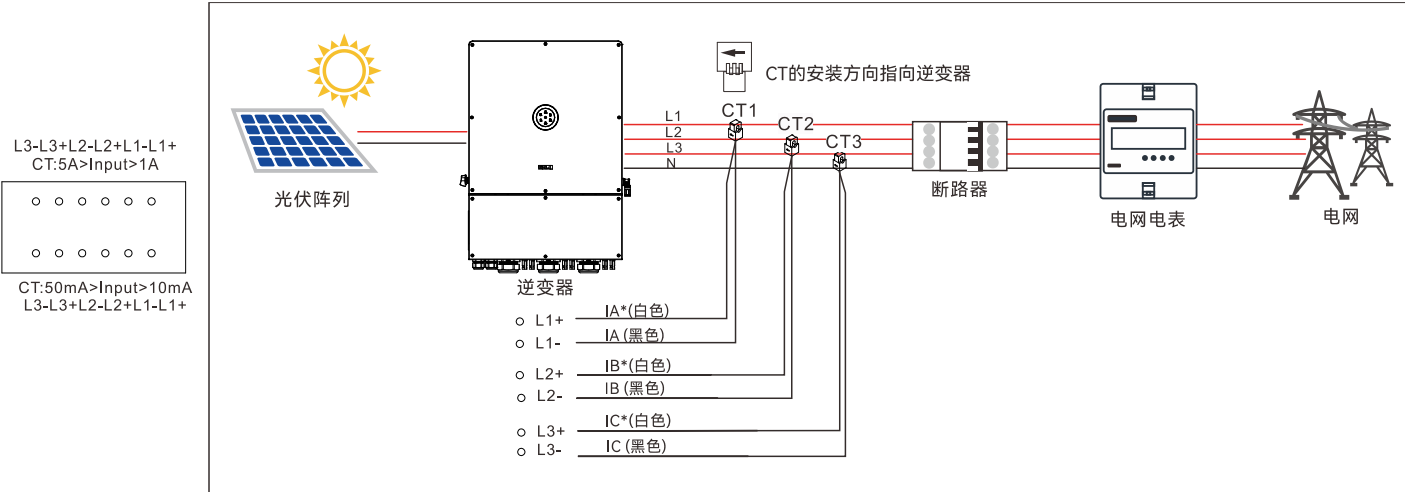
图 5.8. 电网电流互感器连接
