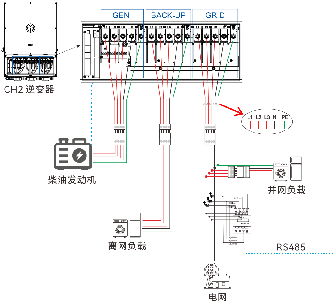
图 5.38. 单台设备部署的系统连接（带离网负载和并网负载）
