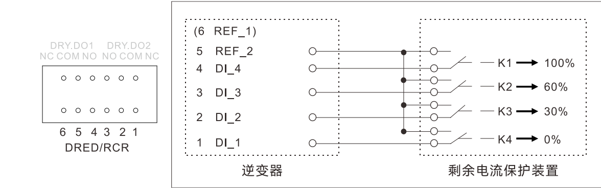
图 5.17. RCD 连接
