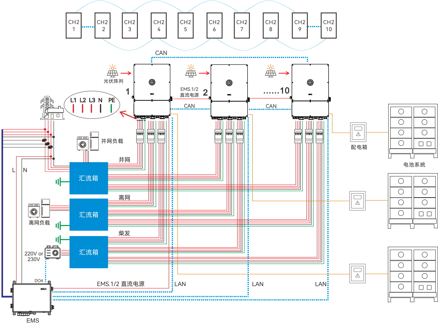
图 5.40. 并机部署的系统连接（离网负载与并网负载）
