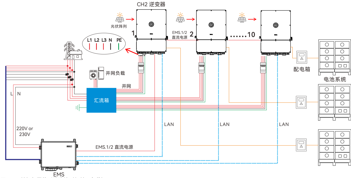
图 5.42. 并机部署的系统连接（仅并网负载）
