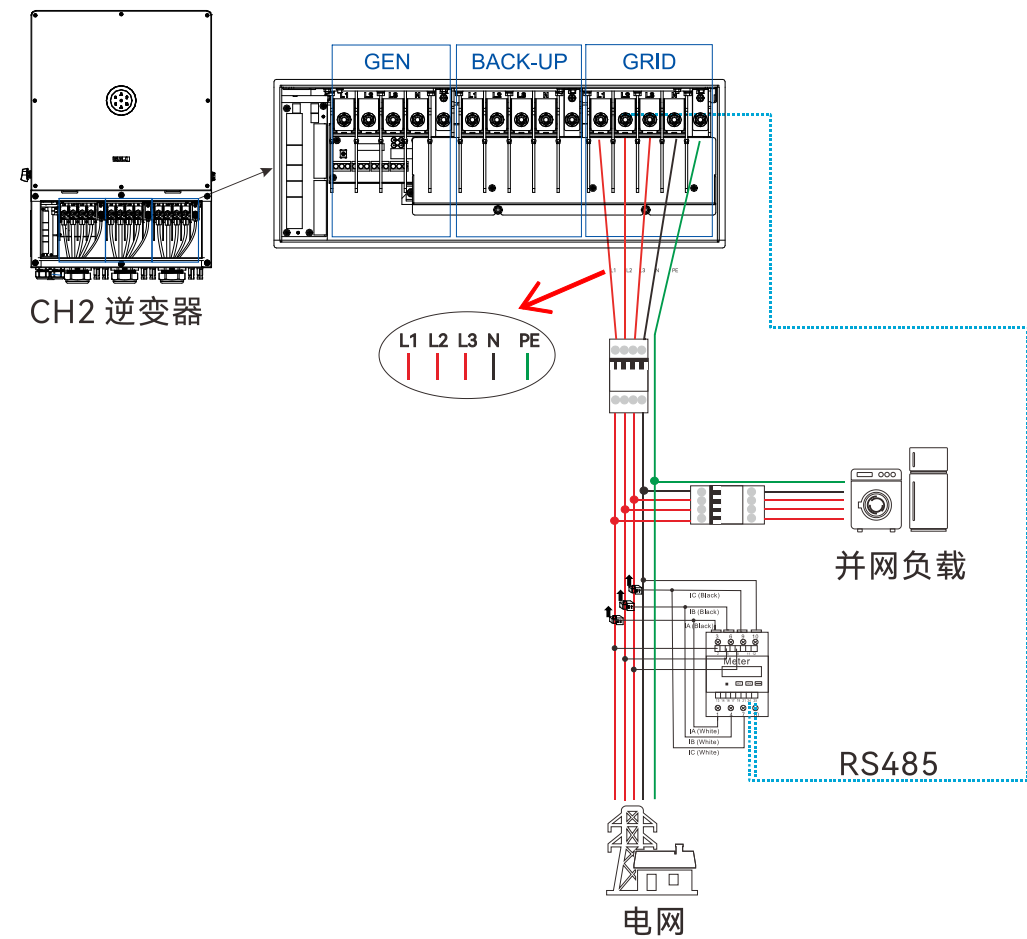
图 5.39. 单台设备部署的系统连接图（仅并网负载）
