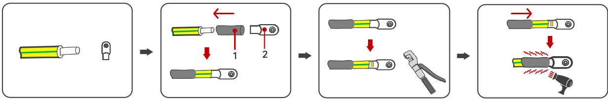
1-Tubo termorretrátil 2-Terminal OT/DT
